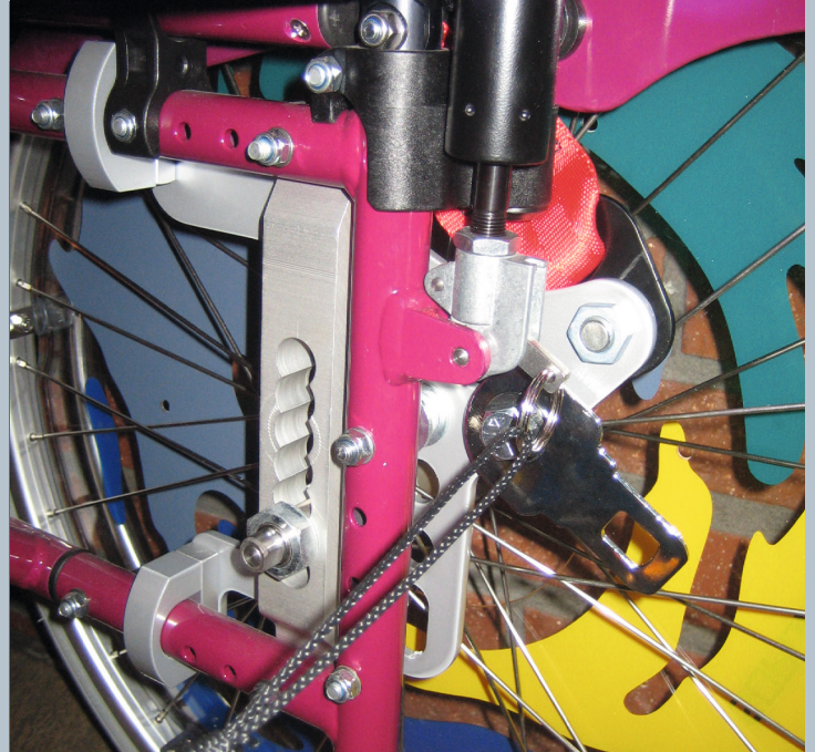
Zwei hintere Kraftknotensysteme mit jeweils einer genormten Schwerlastöse für Spannretractor. Der Beckengurt ist bereits fest montiert.
