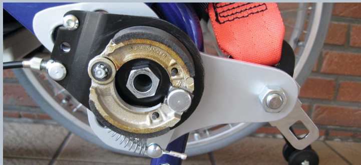
Zwei hintere Kraftknotensysteme mit jeweils einer genormten Schwerlastöse für Spannretraktor. Der Beckengurt ist bereits fest montiert.
