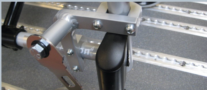
Zwei vordere Kraftknotensysteme mit jeweils einer Schwerlastöse für Spannretractor oder Statigurt.
