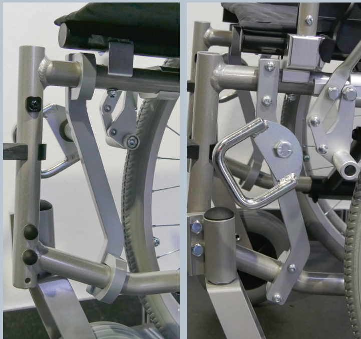
Zwei vordere Kraftknotensysteme mit jeweils einer Schwerlastöse für Spannretraktor oder Statikgurt.
