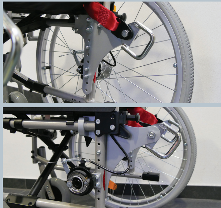
Zwei hintere Kraftknotensysteme mit jeweils einer genormten Schwerlastöse für Spannretraktor. Der Beckengurt ist bereits fest montiert.
